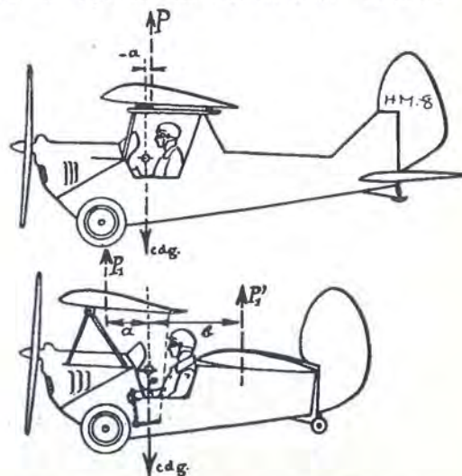
Øverst en Flyvemaskine af sædvanlig Type. Nederst „Pou«en» med de to Bæreplaner, der giver større Frihed i Valget af Tyngdepunktets Beliggenhed.
