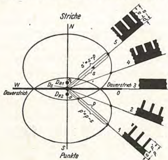
Reflektorerne DR1 og DR2 frembringer i den underste Kurve en Priklinie og i den øverste Kurve en Streglinie.
