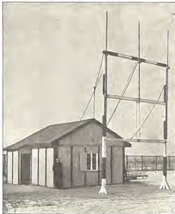
Fig. 1. Forsøgs-Landebaaken paa Tempelhof ved Berlin.
