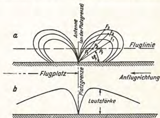
Vertikalkarakteristik af en lodret Dipol. Skitsen viser, hvorledes Lydstyrken efterhaanden tiltager i Nærheden af Sendedipolen for at falde til Nul umiddelbart over denne.
