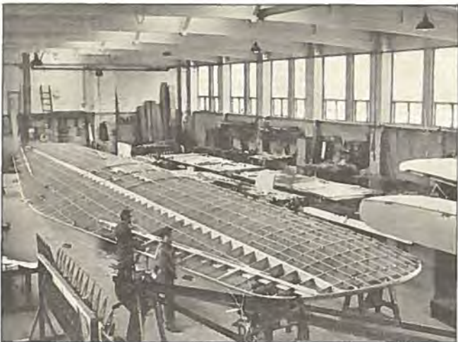
1 1/2 — Den færdige Plankonstruktion.
