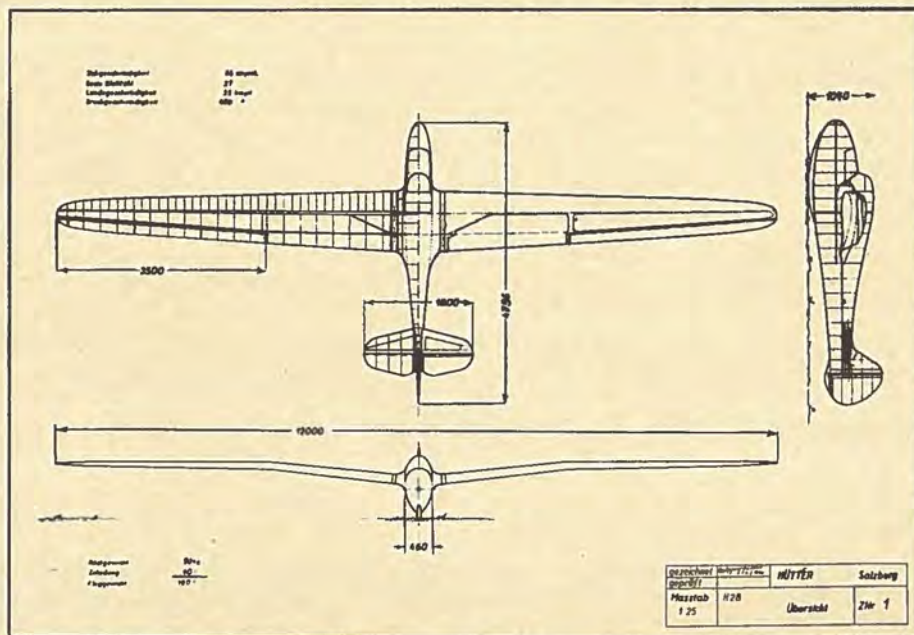
Planbygning for H 28.
