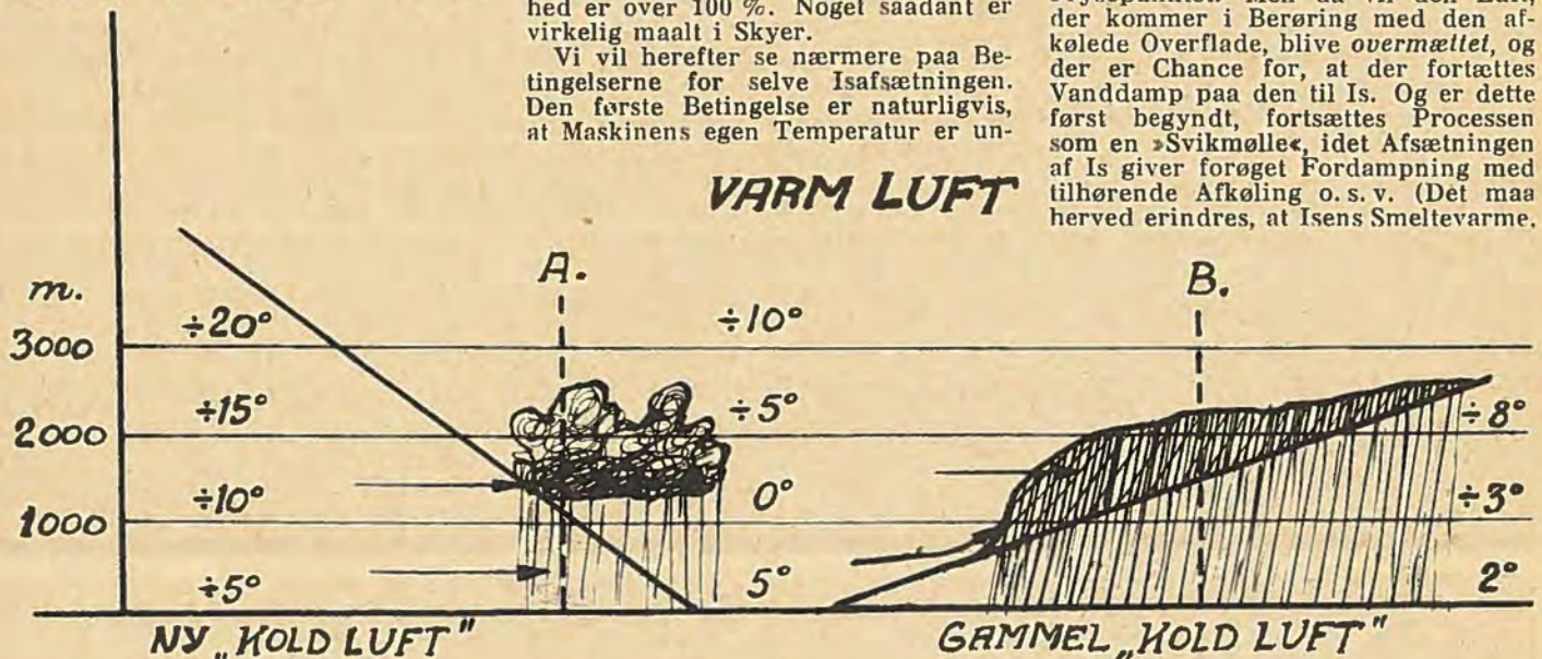
Fig. 2. Tværsnit af »Koldfront« (til venstre) og »Varmfront« (til højre).
