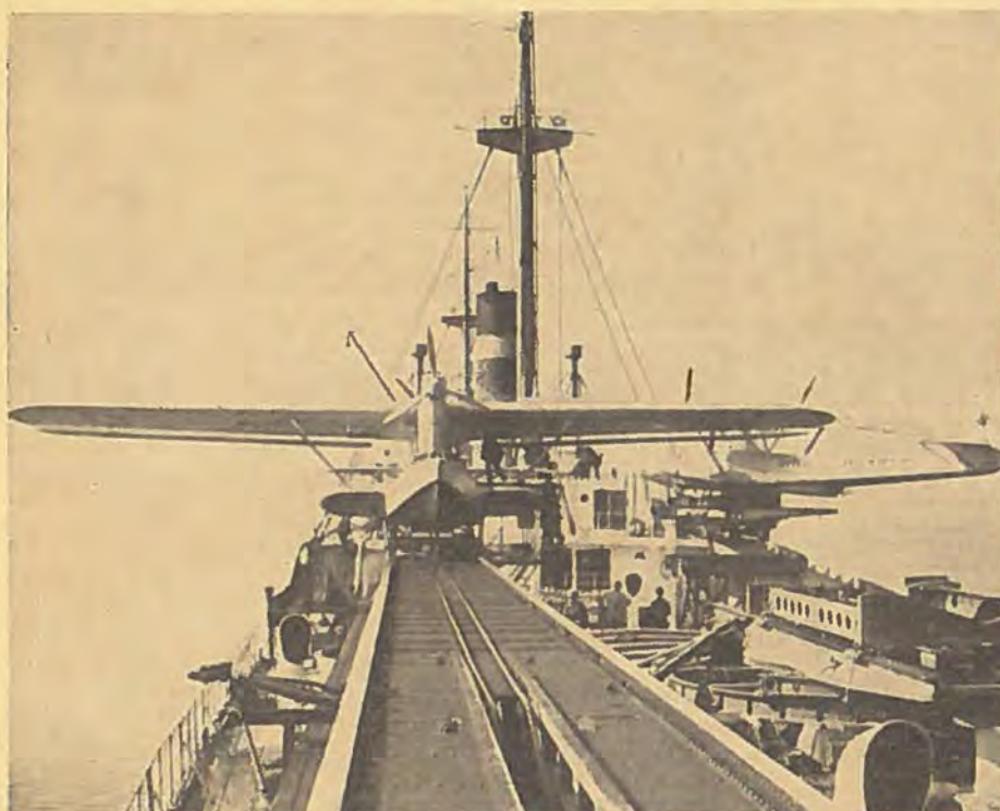
Katapultanlægget paa »Schwabenland«.
