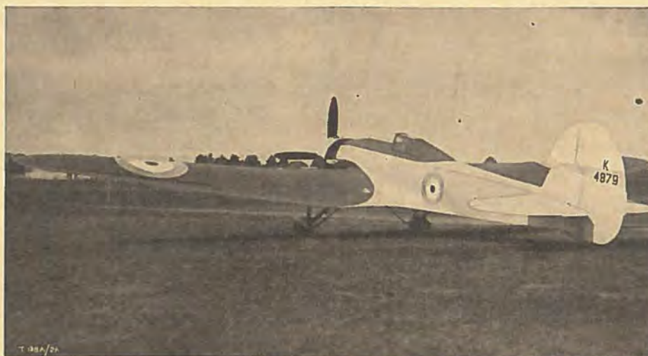
Bristol 138 a — et eensædet Monoplan med en Spændvidde paa 22 Meter.
