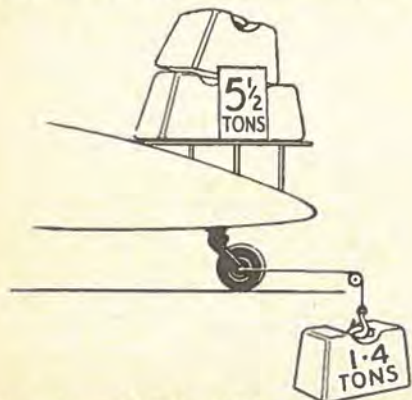
Den bageste Del af Kroppen og Halehjulet kan bære en Belastning paa 5½ Tons og samtidig staa for et Træk bagud paa 1,4 Tons.
