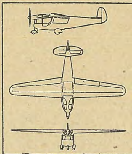
Den svejtsiske Sportsmaskine Farner W. F. 12.
