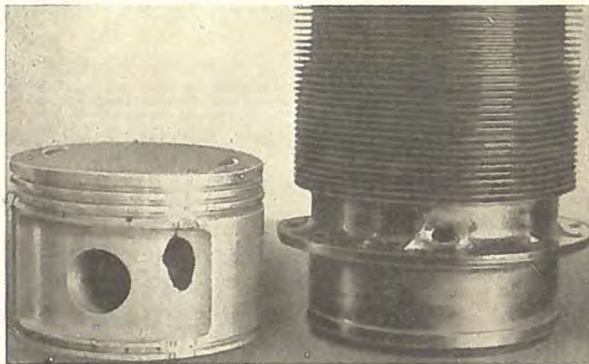
Fig. 6. Gennemskudt Cylinder og Stempel fra den i Teksten omtalte Motor Bremo 323.
