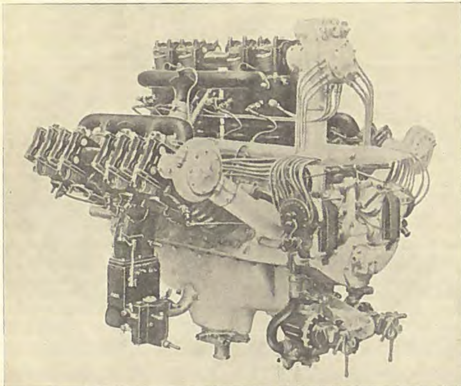
12-cylindret vandkølet Flyvemotor af gammel Type. Motorydelse ca. 450 HK.
