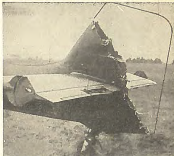
Fig. 5. Finne og Sideror bortskudt paa en Ju 87. Den indtegnede sorte Kontur viser, hvortledes Halepartiet normalt ser ud. Maskinen returnerede ved egen Hjælp.
