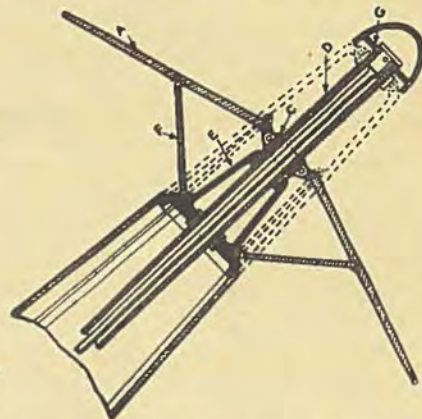
Skitsen viser Dykbremsen, naar den er i Stilling og de punkterede Streger viser den sammenklappet.
