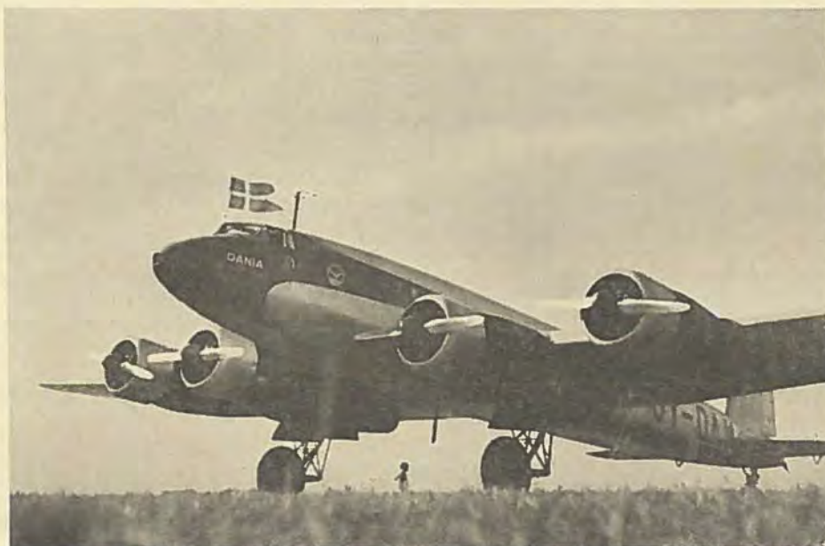
Focke-Wulf Fw 200 »Condor«. Helmetal-Luftfartøjer. Købt ved Fabriken i Tyskland 1938. 4 \times 720 HK. BMW 132-G Motorer. 4 Mands Besætning og 26 Passagerer. Indtrækkeligt Understel. Marchhastighed 330 km/T.
