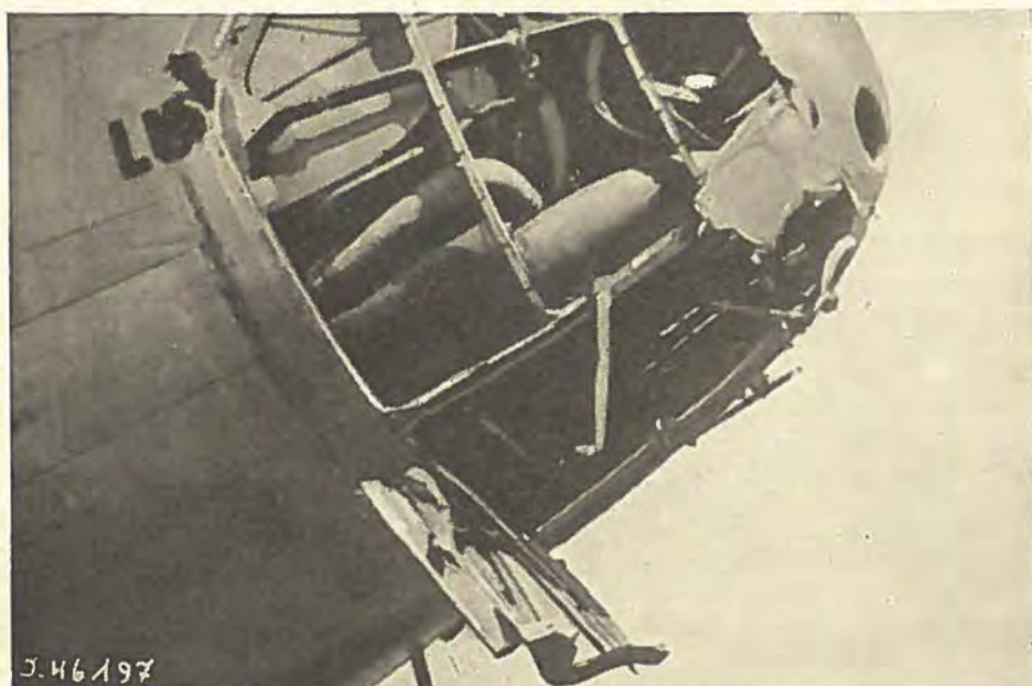
Den forreste Del af Næsen paa en Ju 90 er blevet beskadiget ved Lynnedslag.
