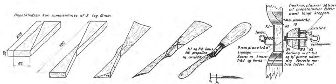
Fremstilling af propel som vist på Kongsberg-tegningen.
