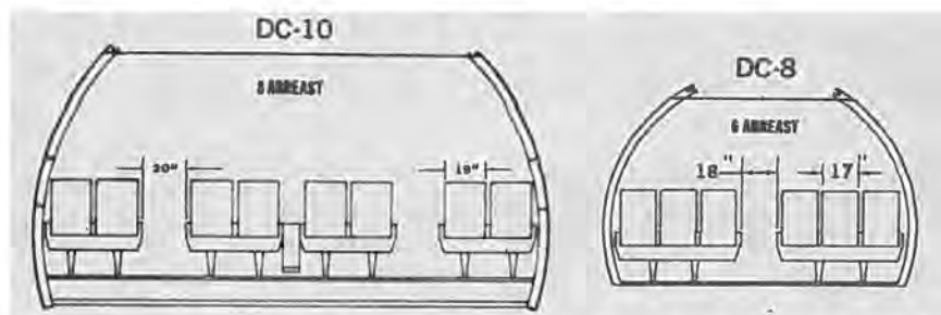
Tværnsnit af DC-10 og DC-8.
