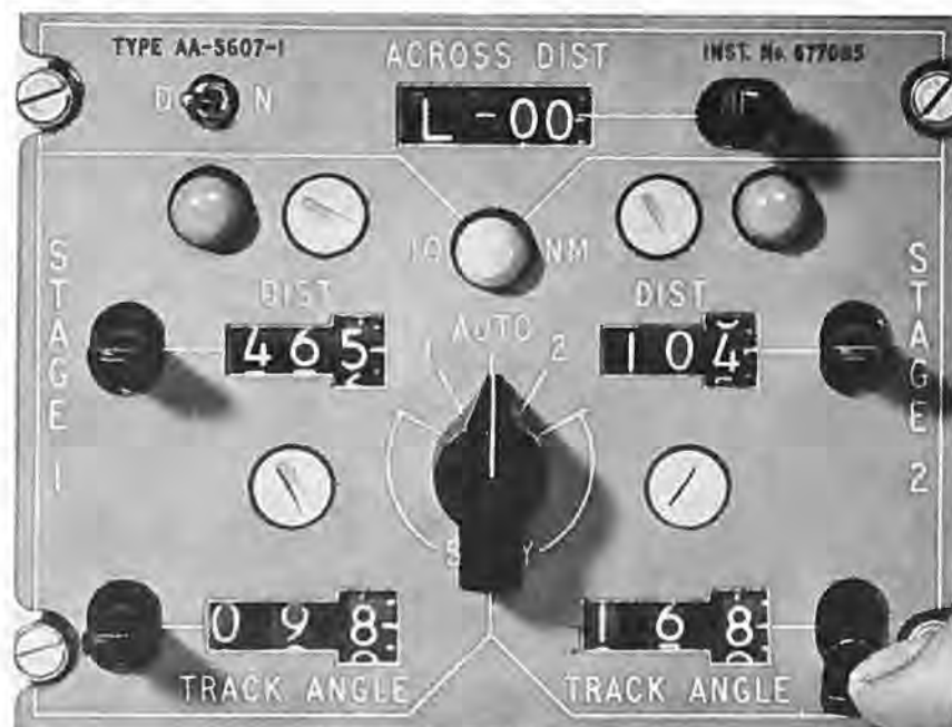
AD-560'ens panel indstillet til brug med autopilot, så den selv skifter over fra det ene ben til det næste, når vendepunktet passerer.
