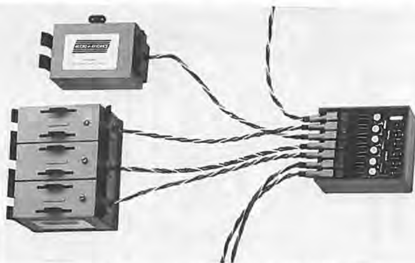
Ledningerne til rormaskinerne tilkobles med stik inde i modtageren. Når låget sættes på denne, er stikkene låst fast.
