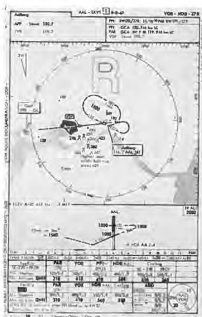
Anflyvningskort for Ålborg.
