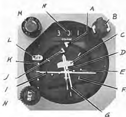
R-1 Pictorial Deviation Indicator til VOR/LOC
