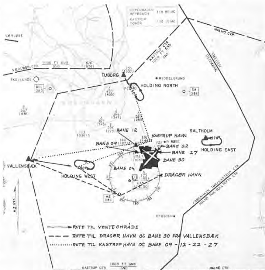
Hvordan man normalt fra rapportpunkterne Vallengsbæk og Tuborg — eventuelt via venteområderne — dirigeres til de forskellige landingsbaner.
