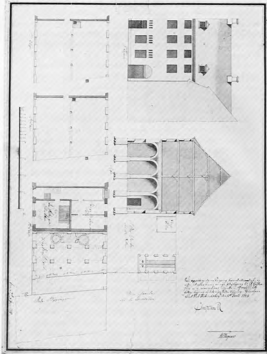
Fig. 24. Forbindelsesbygningen 1789. Nationalmuseets billedarkiv.
