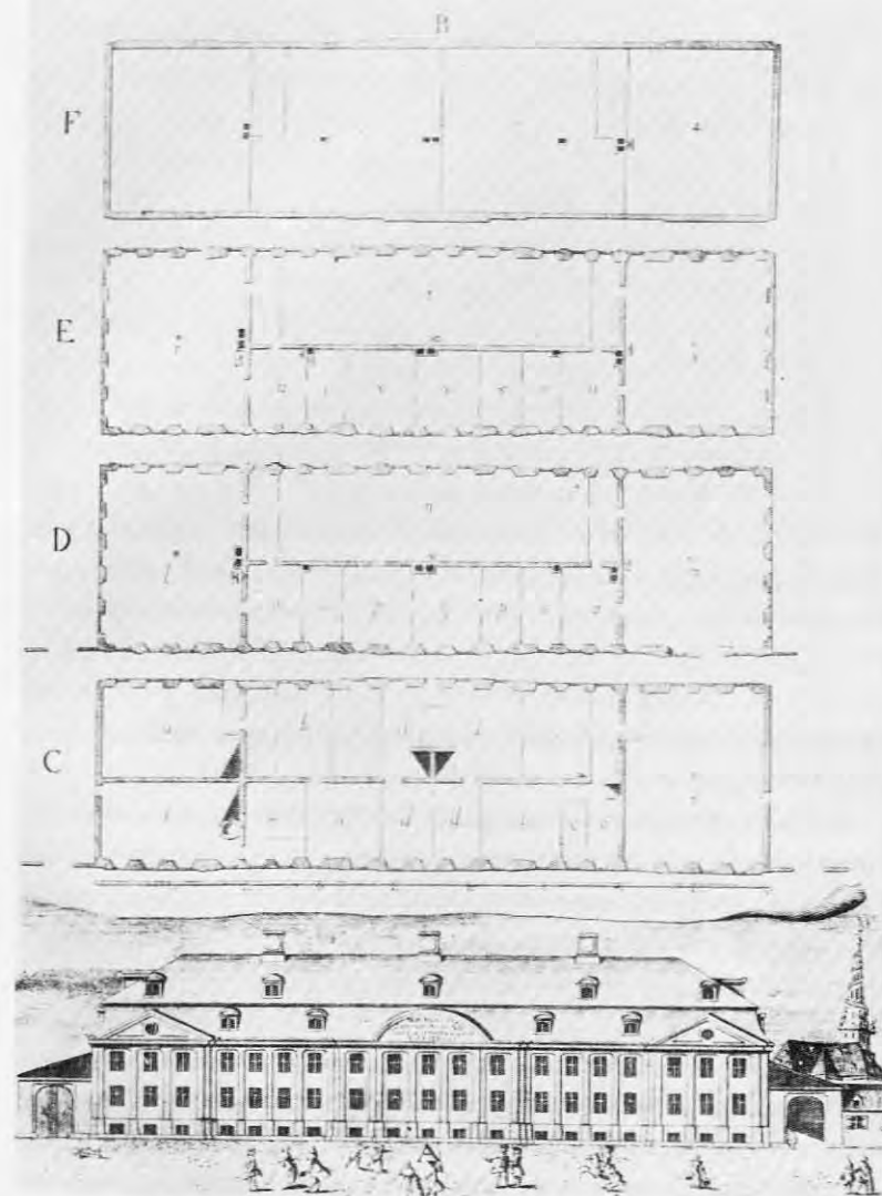
Fig. 20. »Det kongelige stiftede fattige børns Opfostrings-Huus paa Christianshavn«. Stik af G. W. Baurenfeind 1753 34 .
