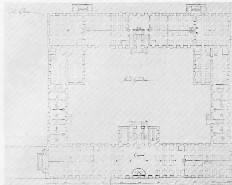
Fig. 18. »Grundtegning af Plan til Qvest-Huus til 1500 Mand, første Etage«.
