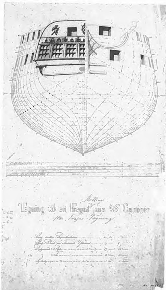
Konstruktionstegningerne til fregatten "Bellona", hvorpå er indtegnet ændringer i apteringen foretaget med henblik på skibets togt til Sydamerika 1840-41. (Rigsarkivet).
