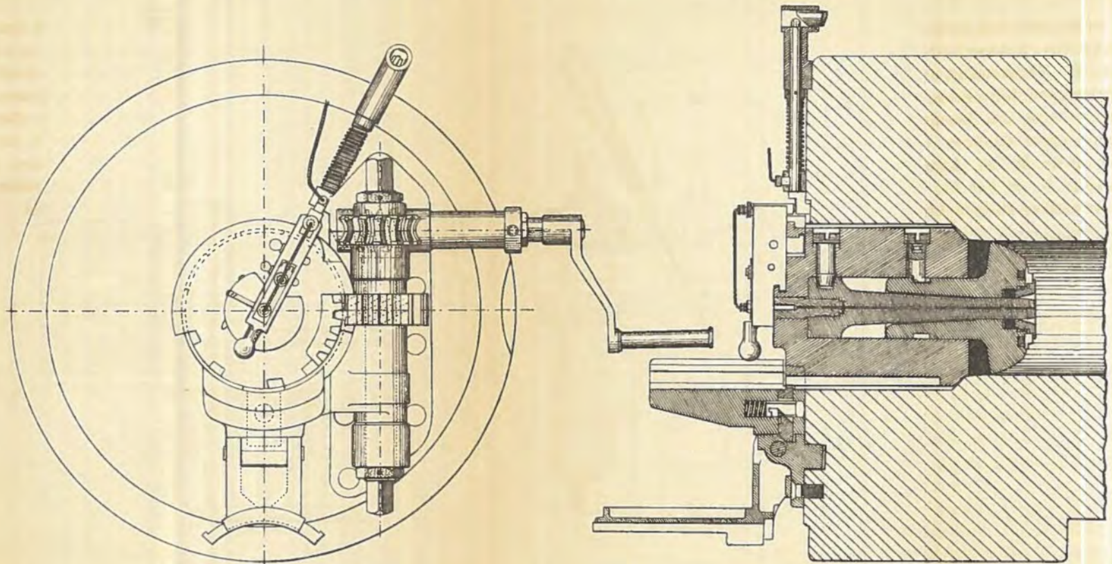
Canets Skruemeckanisme til 24 \frac{c}{m} B. K.
