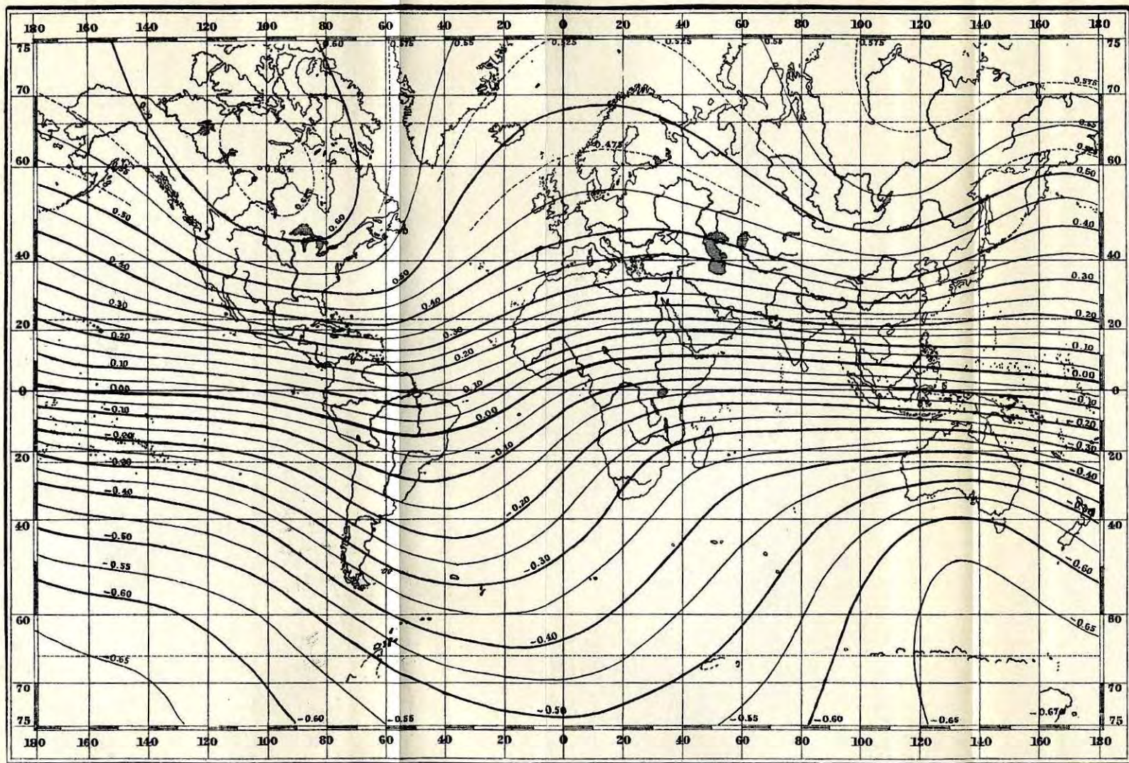
Figur 3 Kort over Vertikal-Intensiteten ved Dr. Adolf Schmidt. 1885. O. —
