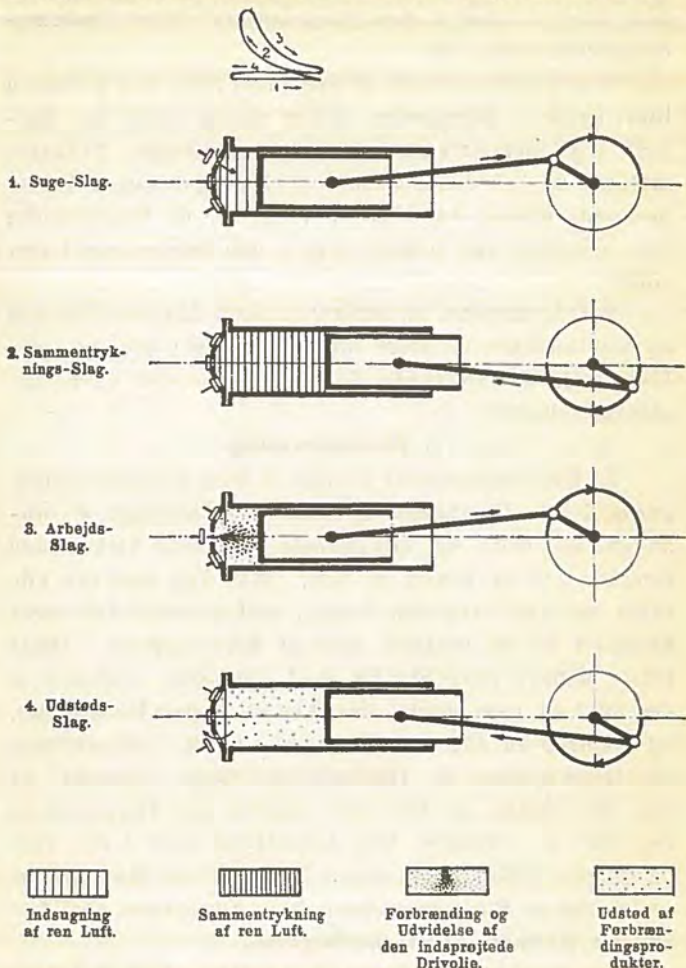
Fig. 2. En 4-Taksmotors Virkemaade.
