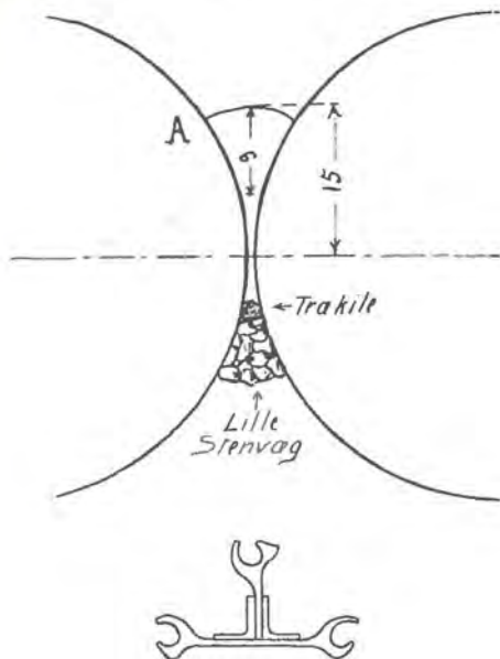
Fig. 8. Cylinderforbindelsen.
