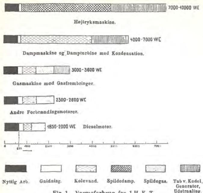
Fig. 1. Varmeforbrug for 1 H. K. T. (Efter M. A. N. Dieselmotoren).
