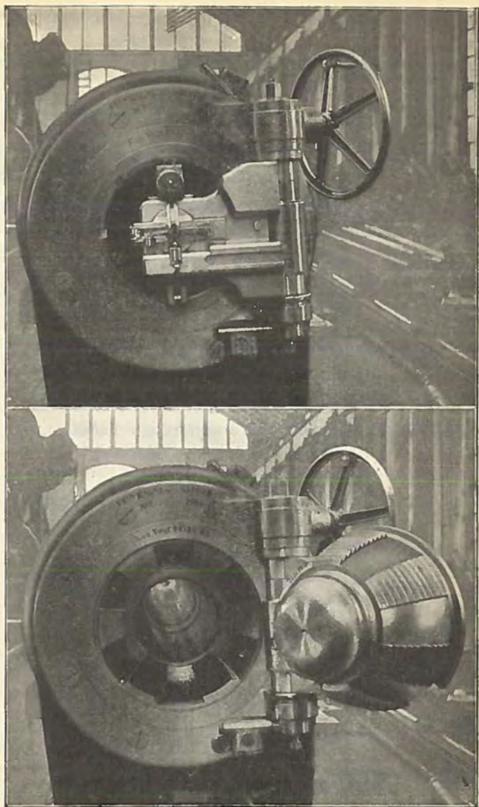
Fig. 5. Bofors Baglademekanisme (24 cm. K. L/48).
