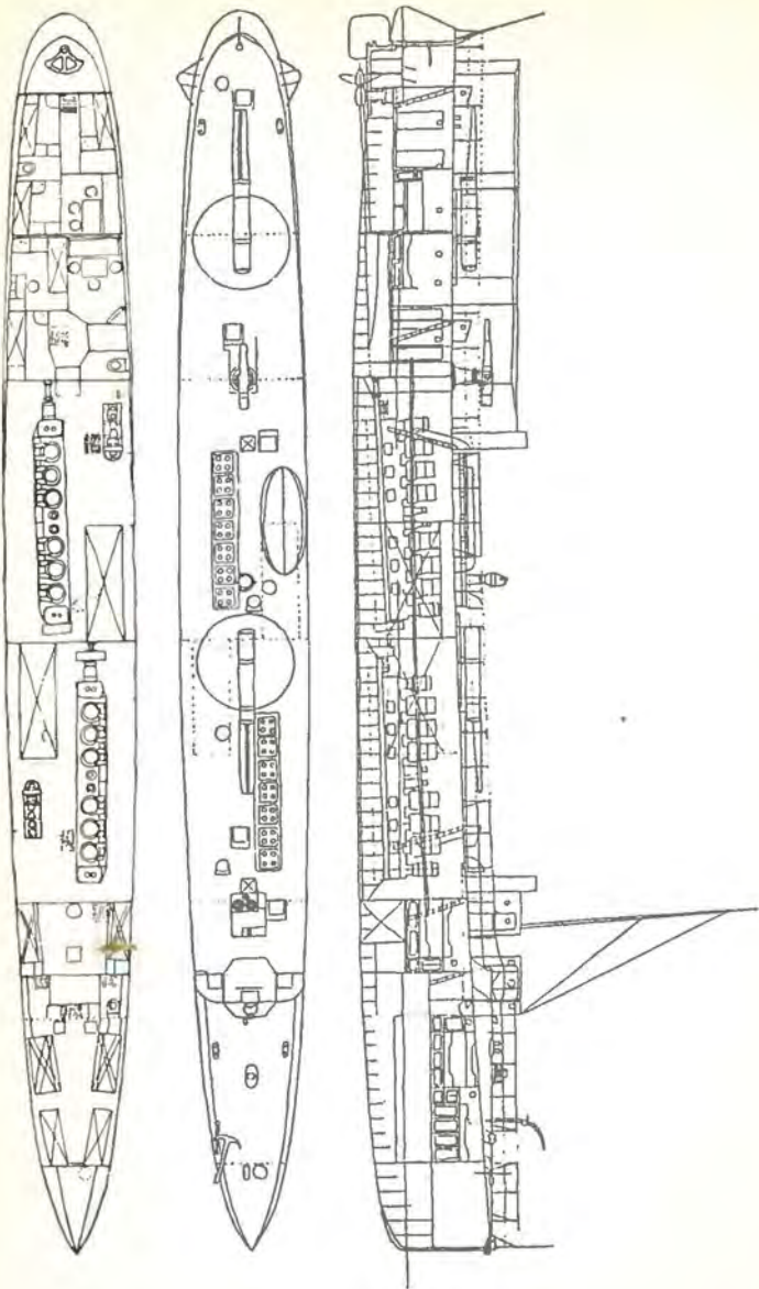
Fig. 9. Germanlavertfels Udkast til en 125 Tons Motortorpedobaad.
