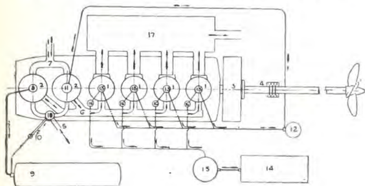
Fig. 3. Skematisk Tegning af en Marine-Polar-Motor. (Efter Schiffbau.)
