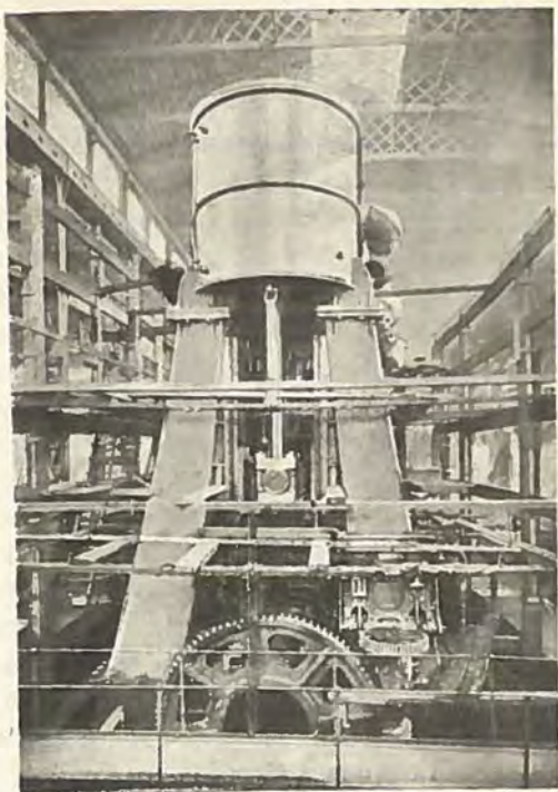
Styrbords Stempelmaskine, set agterfra.
