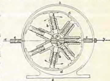
Fig 2. Indstrømning gennem p. Udstømning gennem q.
