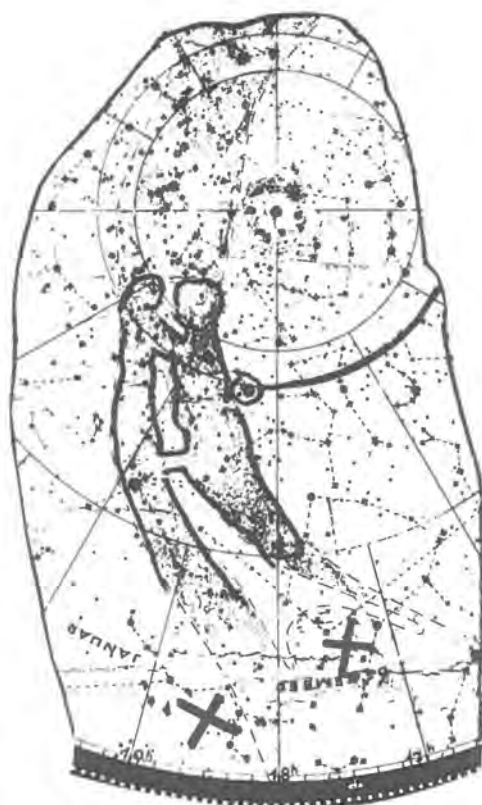
Fig. 15. Stjernerort. Den sydlige himmel til solhverv.
