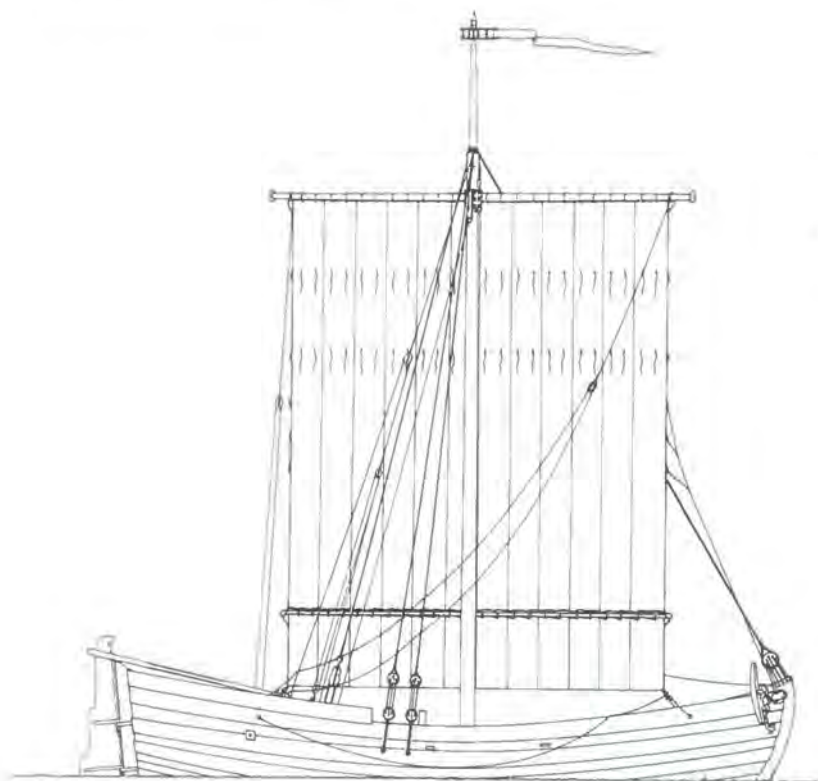
Rekonstruktion af sandskuden fra Klim Strand. Tegning: Morten Gothche.
