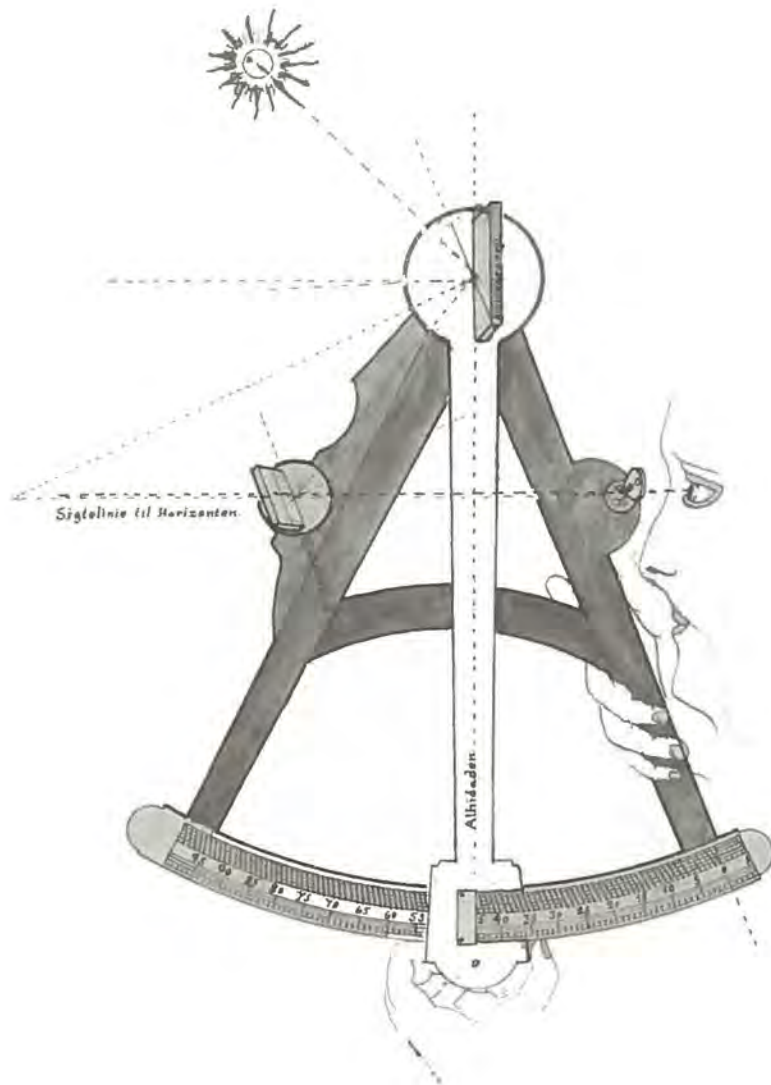
Figur 62. Højdemaaing. Spejloktaten. Alhidadespejlet og Horizontspejlet skal staa lodrette paa Instrumen- tets Plan og være parallelle naar Instrumentet staaar paa o. Opfun- det af Astronomen John Hadley i 1731.
