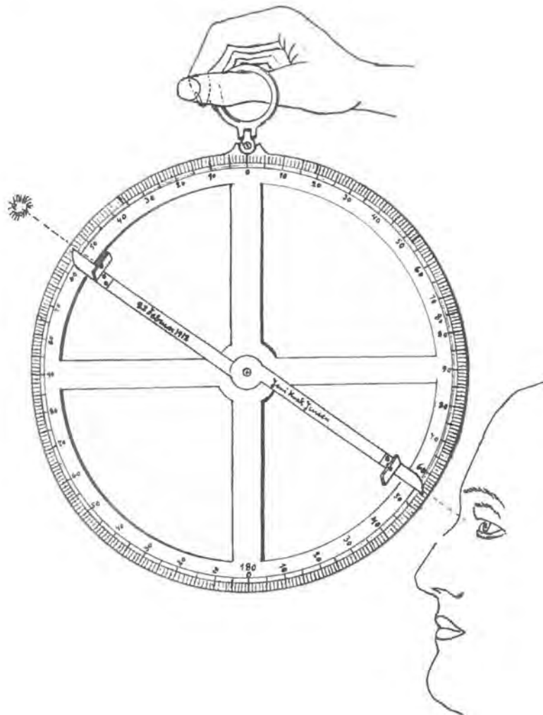
Figur 8. Højdemaaling med Astrolabiet.
