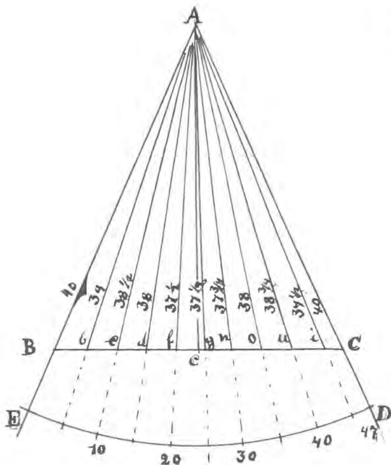
Figur 45. Storcirkelberegning mellem Steder med samme geografiske Bredde.
