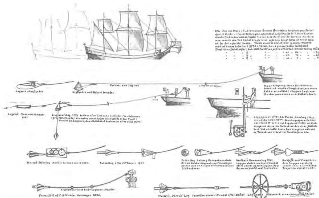
Figur 29. Bestemmelse af Skibets Fart.
