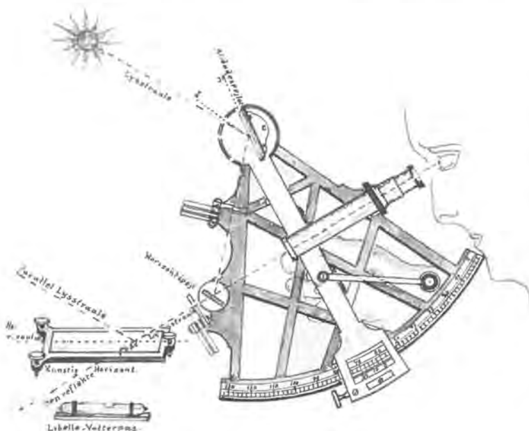
Figur 68. Maaling med Sekstanten over kunstig Horizont. Maaling med Sekstanten over kunstig Horizont. Sekstanten kendt 1790. Vinklen imellem de reflekterede Billeder fra Albidde-spejlet og den kunstige Horizont er dobbelt saa stor, som Højden over den horizontale Linie. Den kunstige Horizont kan bestaa af et Spejl, der stilles horisontalt efter Libelle, eller Kviksølv i en Skaal. Sekstanten inddeles ofte til 10 Buesekunder eller 1/12960 Del af Cirkelns Omkreds. Ved Breddeobservation kan Stedets Bredde findes med en nøjagtighed af 2 ÷ 300 Meter.
