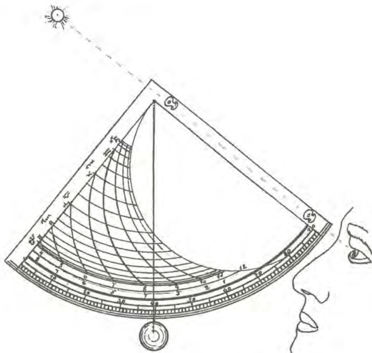
Figur 9. Højdemaaing med Kvadranten.
