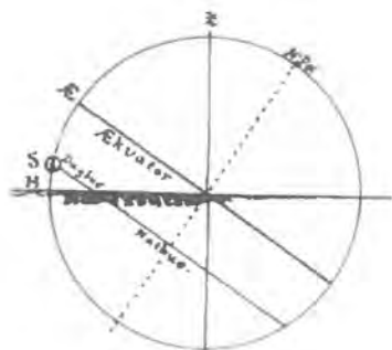
Figur 73. Breddebestemmelse. Bestemmelsen af Stedets Bredde, Afstand fra Ækvator, var i Oldtiden og Middelalderen den vigtigste og mest paalidelige af de astronomiske Observationer, der kunne udføres med Datidens nautiske Instrumenter. Himmellegemets største Højde maalttes naar det stod i Middagsmeridianen.
