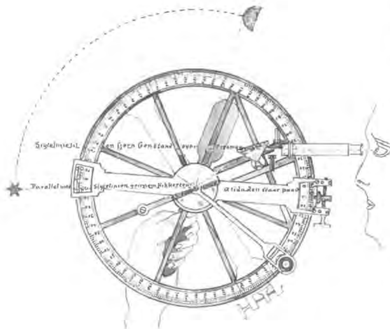
Figur 70. Prismecirklen eller Pistors Cirkel.
