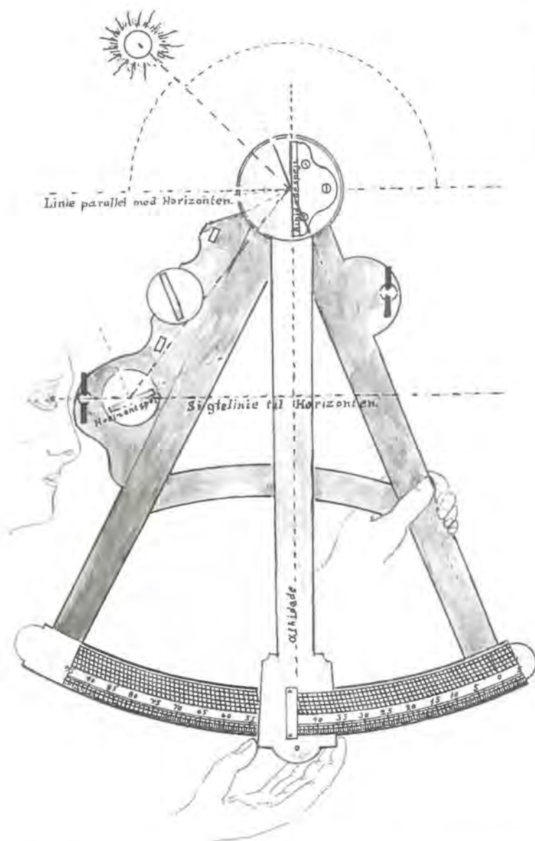
Figur 63. Højdemaaling. Spejloktaten. Fravendt sigte. Alhidadespejlet og Horizontspejlet skal staa lodrette paa Instrumentets Plan og være vinkelrette paa hinanden, naar Instrumentet staar paa 0. Opfundet af Astronomen John Hadley i 1731.
