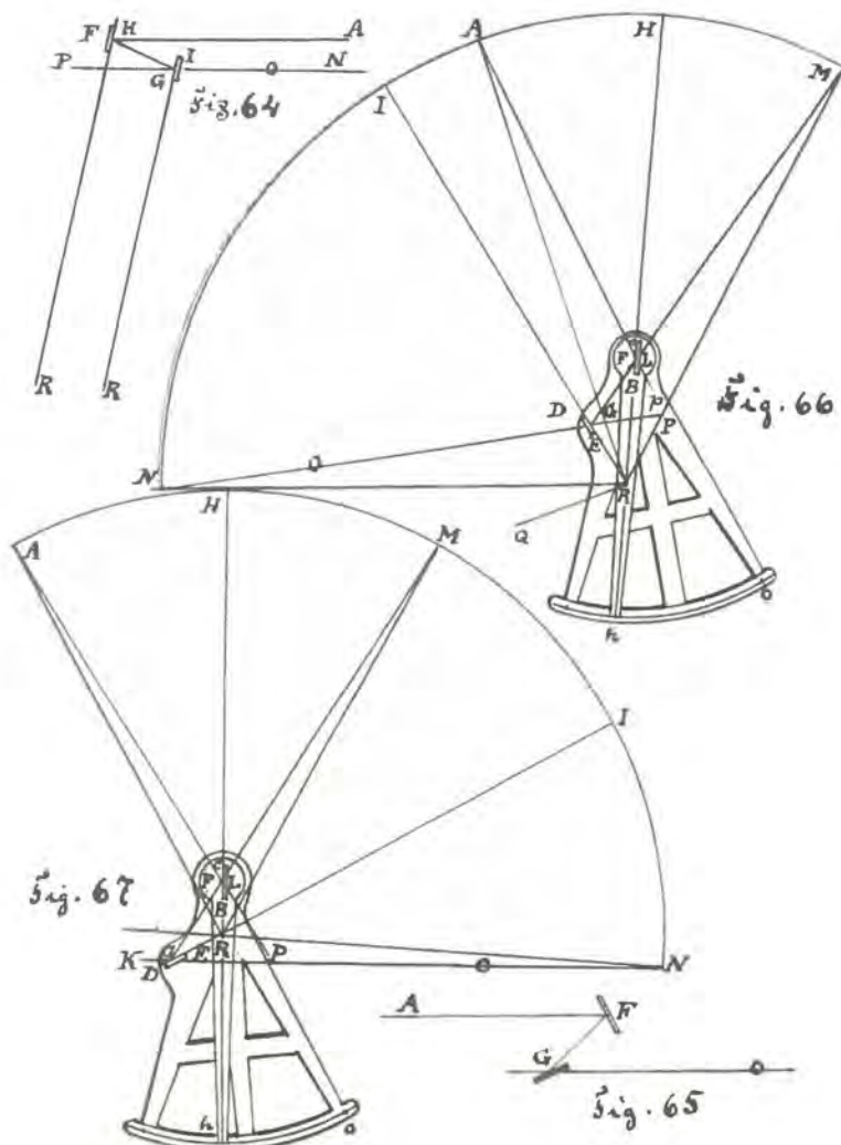
Figur 64-67. Strålegang i Oktanten.
