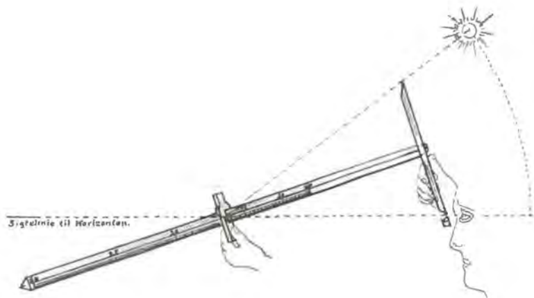
Figur 52. Højdemåaling med den bagvendte Jakobsstav.
