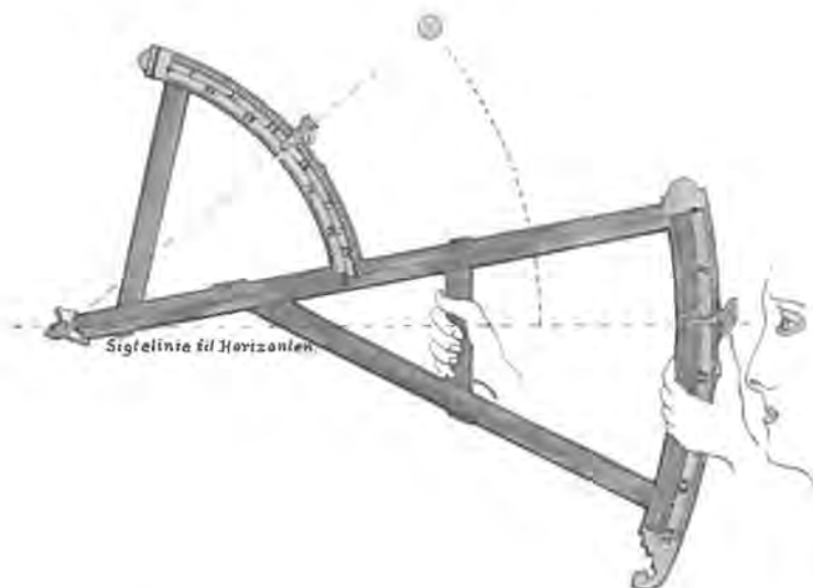
Figur 59. Højdemåling med Davis Kvadrant.
