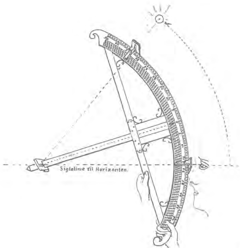
Figur 57. Højdemåling med Cross Bow.
