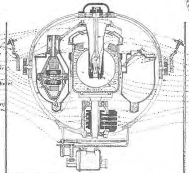
Figur 26. Gyroskop Moderkompas fra Undervandsbaaden »Havfruen« fremstillet af Anschütz.
