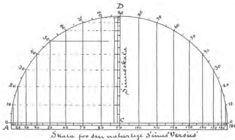
Figur 39. Konstruktion af Sinusskalaen.
