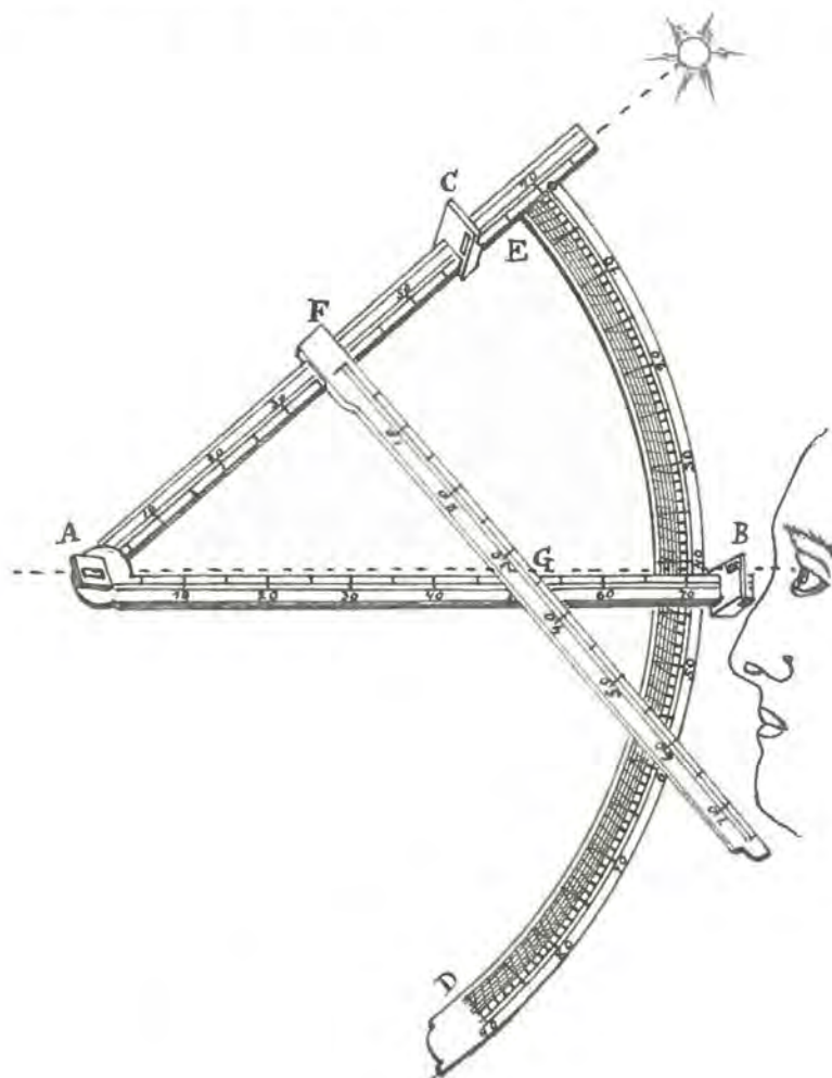
Figur 58. Den Bevægelige Kvadrant.
