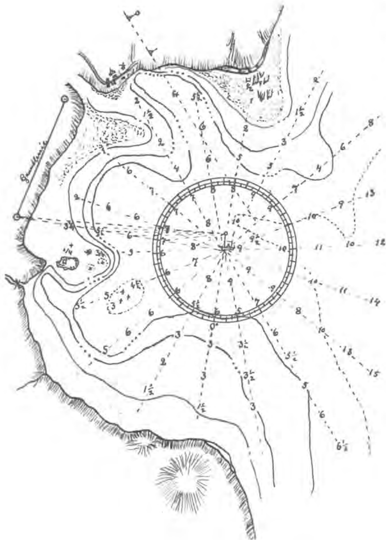
Figur 34. Soopmaaling ved Triangulering fra Grundlinie paa Land.
