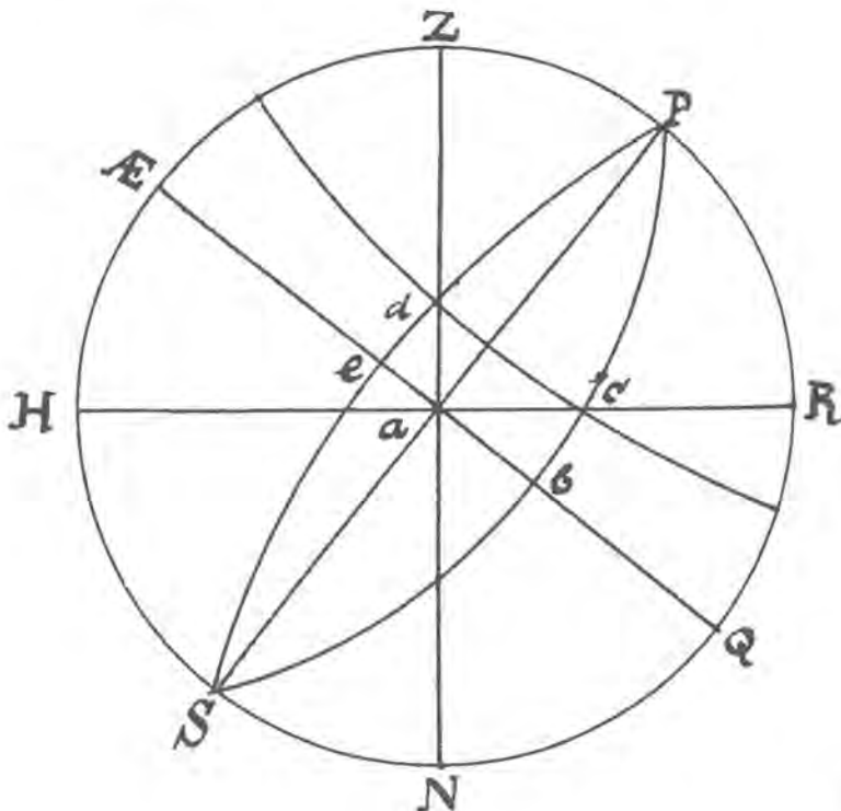
Figur 18. Solens Amplitude.
