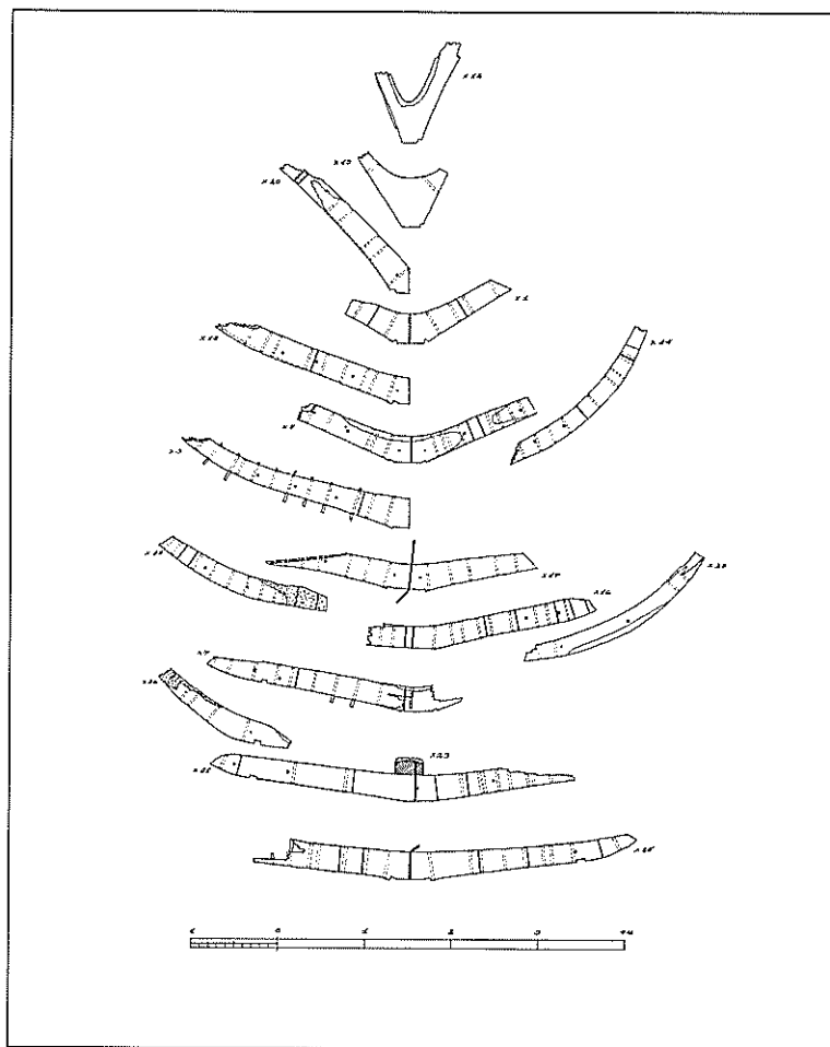
Fig. 3. Opmåling af opgravede spantedelev: bundstokke, sitterser og oplængere. Opmåling og tegning: Morten Gothche, Vikingskibsmuseet i Roskilde.
