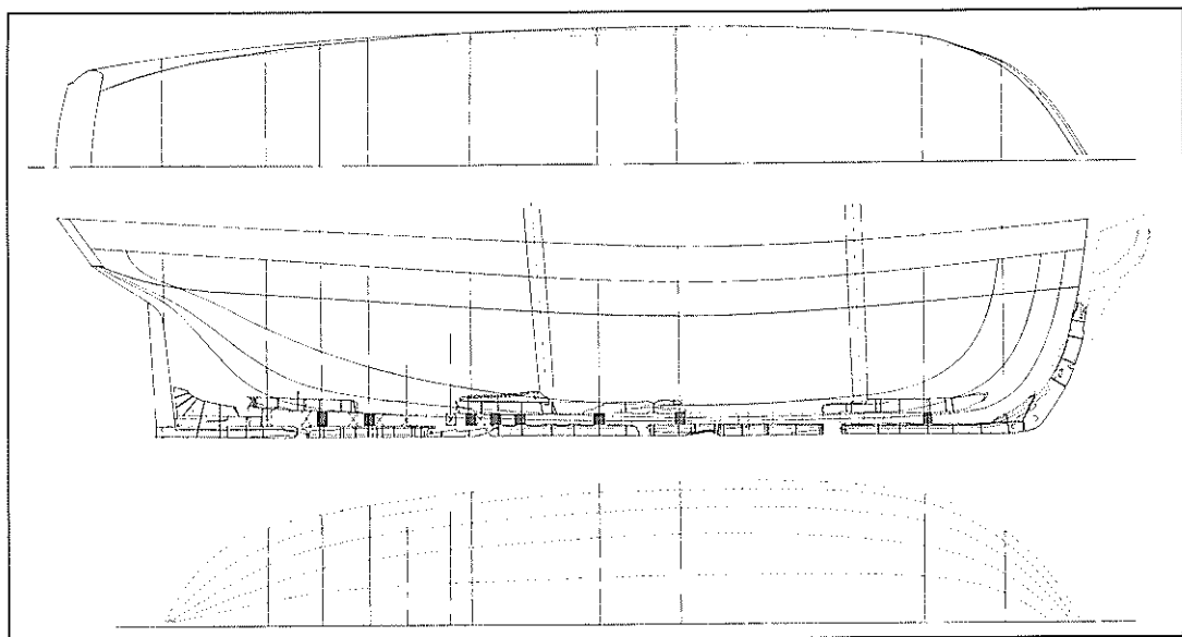
Fig. 10. Rekonstruktion af briggen Anna af Horsens. Skibets hovedmål – længden fra indersiden af forstævnen til spejklædningen agter, bredden mellem tommeret og dybden i lasten – er søgt anvendt ved rekonstruktionen. Rekonstruk- tion: Morten Gothche, Vikingskibsmuseet i Roskilde.
