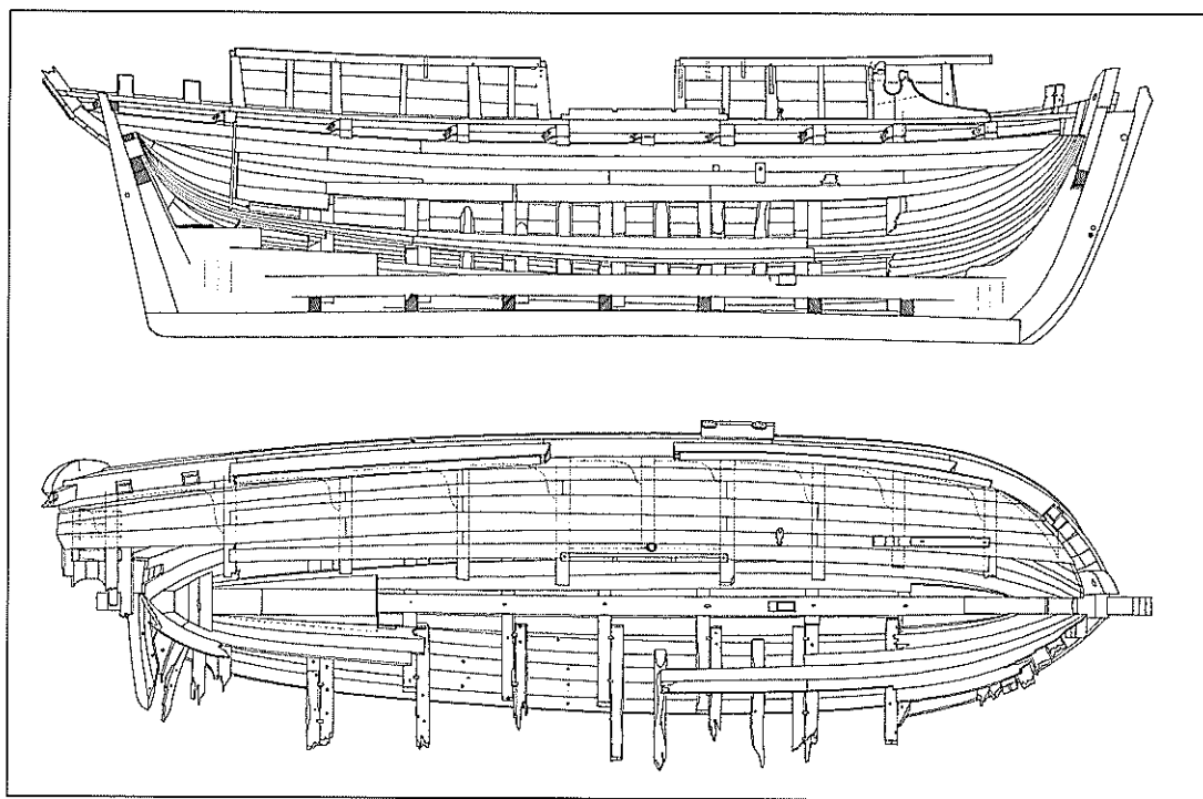
Fig. 5. Uggerbyvrage udgravet af Nationalmuseet i 1984 i samarbejde med Bangsbomuseet. Opmåling: Morten Gothche, Vikingeskibsmuseet i Roskilde.
