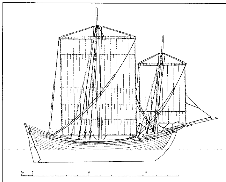
Fig. 8. En rekonstruktion af Bredfjed-skibet. Bemærk de to master og det kraftige spring. (Tegning: Christian Lemée, Vikingskibsmuseet i Roskilde).
