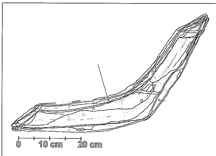
Fig. 4. Stævnknæet. Kaldes også for en bjørn. (Tegning: Morten Ravn, Vikingskibsmuseet i Roskilde).
