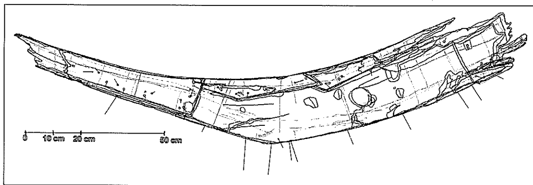
Fig. 2. Stævnloten. Bemærk anlægsfladerne til kolbordet og bordbalsene samt det runde draghul midt på lotens lodrette del. (Tegning: Morten Ravn, Vikingeskibsmuseet i Roskilde).
