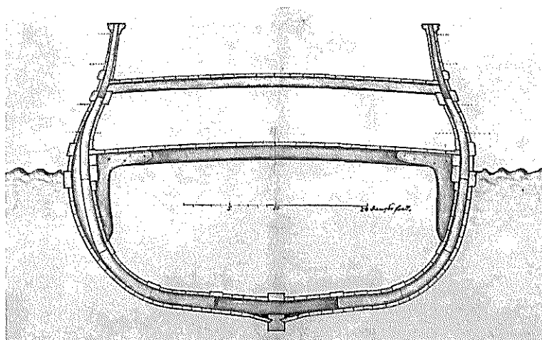
Fig. 12. Dannebrogens mid- delspant. Den påsatte bug ses i bagbordsside. Efter Bjerg & Erichsen 1980 p. 18.
