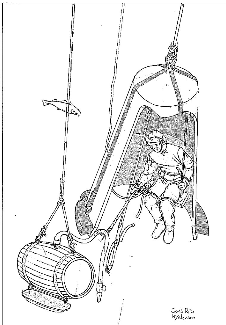
Fig. 1. 1700-tals dykker i dykkerklokke modtager et tilskud af luft i en tønne. (Forf.s rekonstruktion på grundlag af »Konsten af Lefwa under Watn« og Francesco Negris beskrivelse af bjergningsarbejderne fra Vasa).
