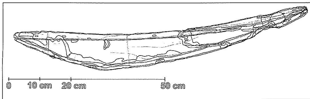
Fig. 6. Stævnikrigen. Øverst ses den flade, der har ligget ind til forstævnen. (Tegning: Morten Ravn, Vikingeskibsmuseet i Roskilde).
