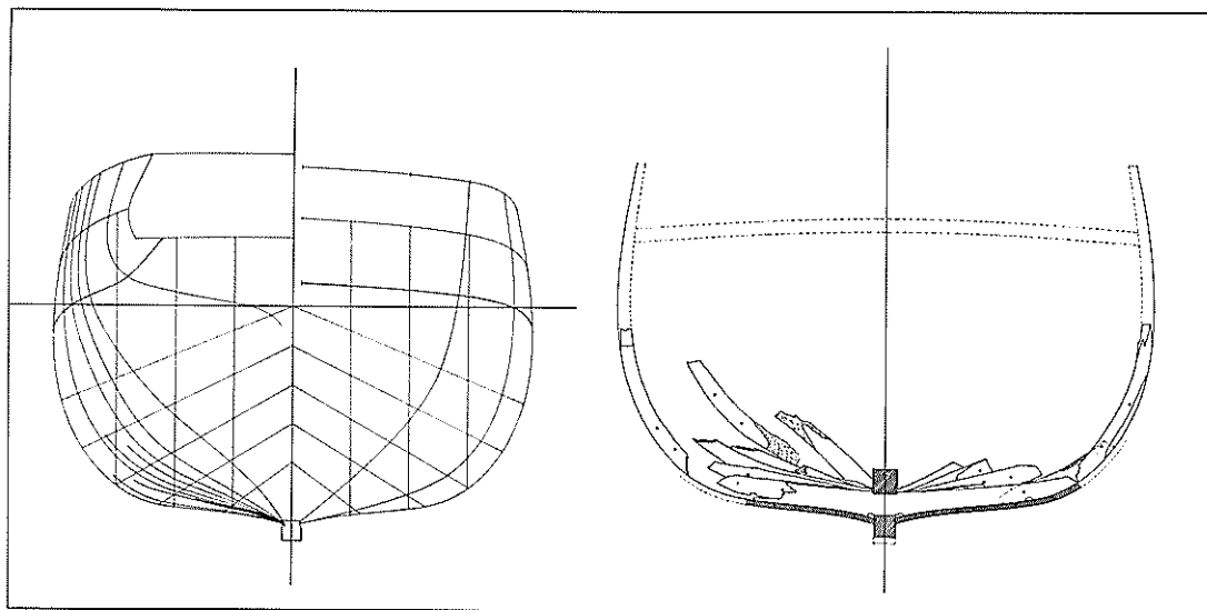
Fig. 11. Rekonstruktion af briggen Anna af Horsens' spanterids og middelspant. Rekonstruktion: Morten Gothche, Vikingeskibsmuseet i Roskilde.
