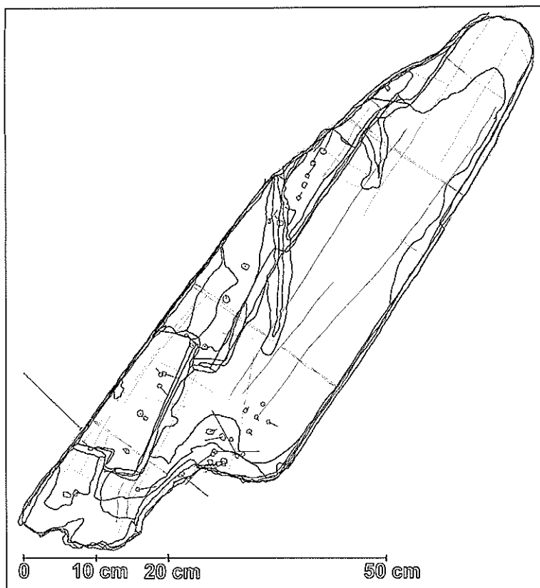
Fig. 3. Agterstævnen. Bemærk anlægsfladerne til bordbalsene og de mange spirhuller til højre på stævnen, der formentlig stammer fra fastholdelsen af rorbeslaget. (Tegning: Morten Ravn, Vikingskibsmuseet i Roskilde).
