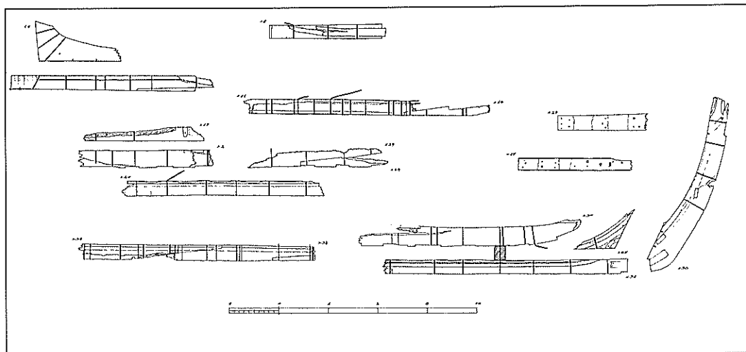
Fig. 2. Opmåling af de opgravede køl- og kølsvinsdele, forstævn med mere. Opmåling og tegning: Morten Gotbche, Vikingeskibsmuseet i Roskilde.
