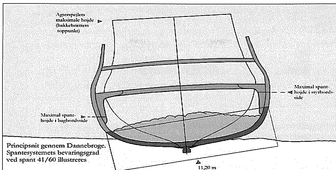
Fig. 7. Principsnit gennem Dannebrog. Ifølge AIS Em. Z. Svitzers oplysninger var vraget bevaret i et ca. 1 m højt niveau i 1873-1875 end i dag. Tegning: J. Christoffersen 1988. Rentegning: Forf. 2004.
