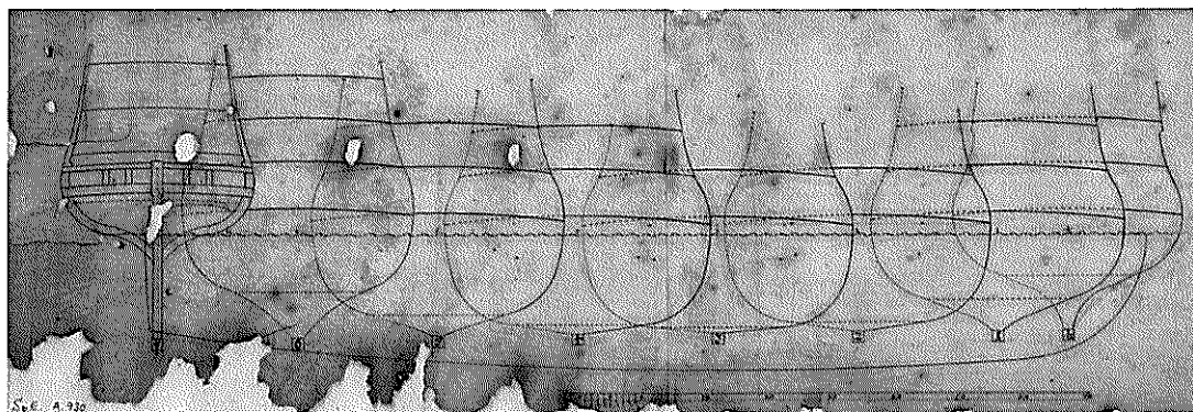
Fig. 18. Dannebrogens spante- rids. Rigsarkivet Des. A930.
