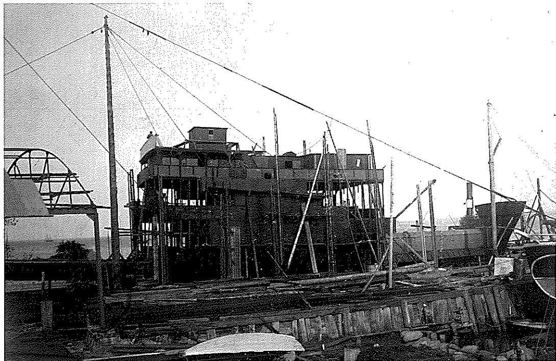
s/s ENIGHEDEN 1917 under opbygning på H. C. Christensens værft. Foto: Marstal Søfartsmuseums Arkiv.
