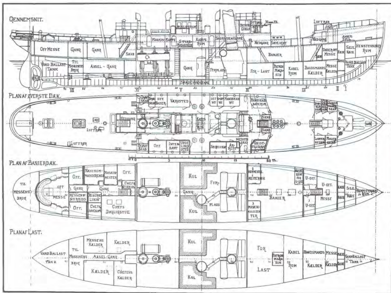
Apteringstegning af inspektionsskibet "Islands Falk", 1906.
