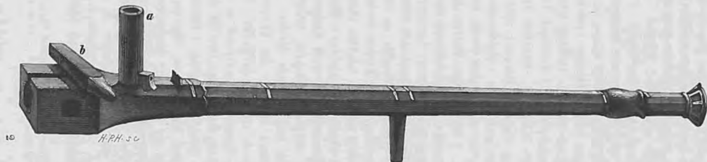
Fig. 3 b. Bagladekanon 2. a løst Kammers (Kammerstykke) af Jern, til Krudtladningen. b Bolt bag Kammerset, naar det er sat helt ind i Løbet.
